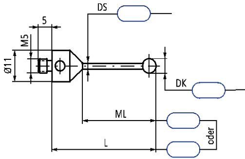
Typ 1: Standard
