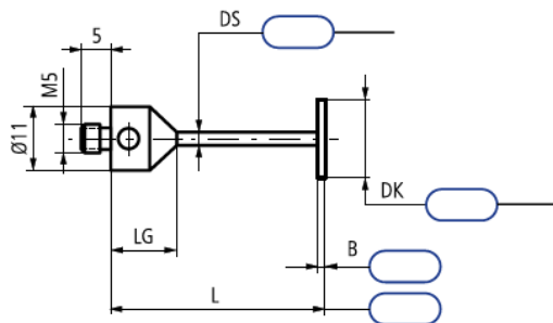
Typ 3: Scheibentaster
