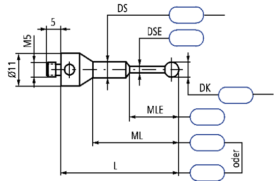
Typ 2: Abgesetzt
