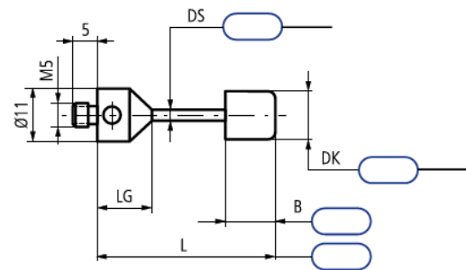
Typ 4: Zylindertaster
