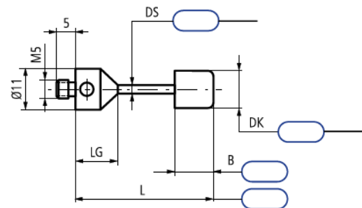
Typ 4: Zylindertaster
