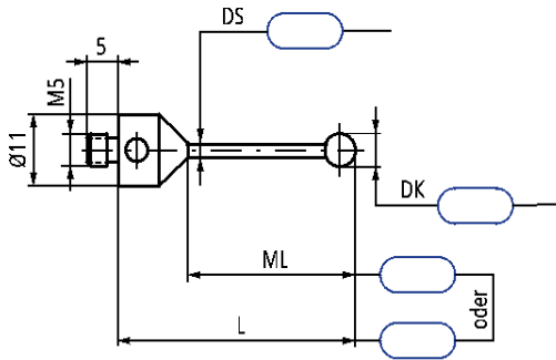
Typ 1: Standard
